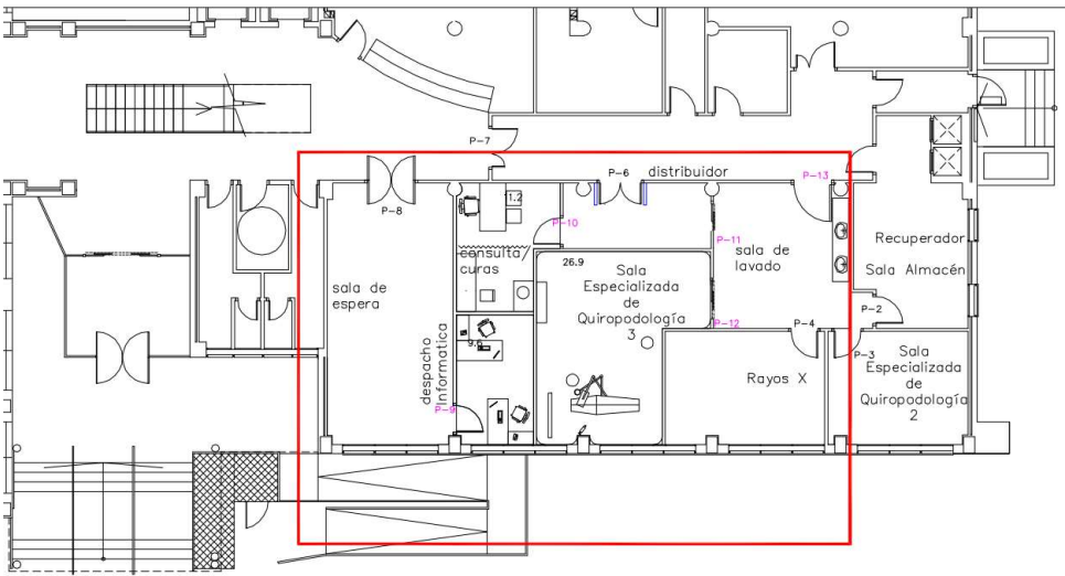
PLANTA BAJA
